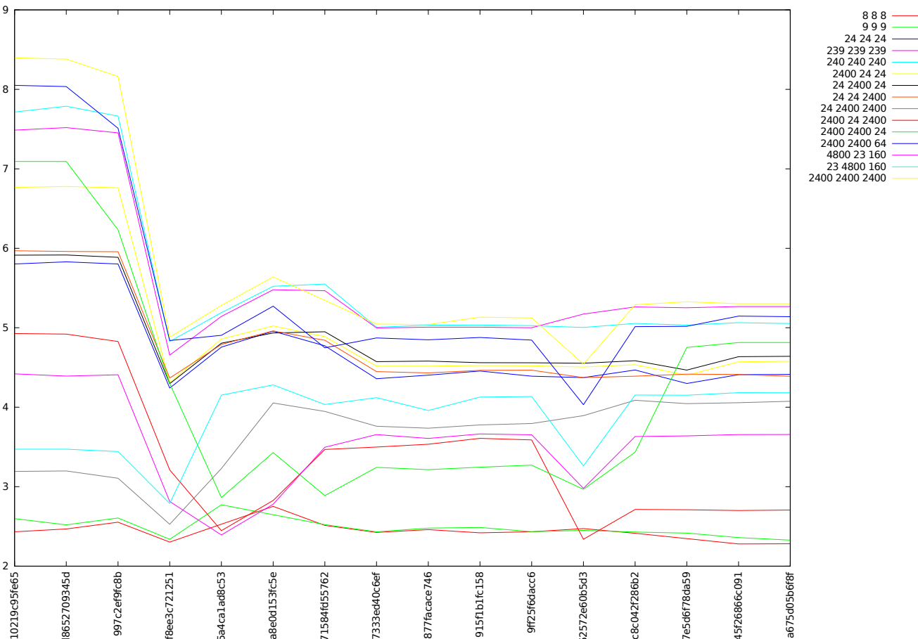
penryn-sse4-dgemm
